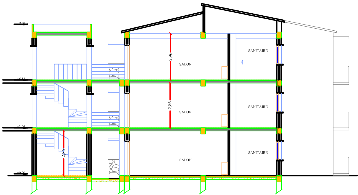
COUPE A-A
