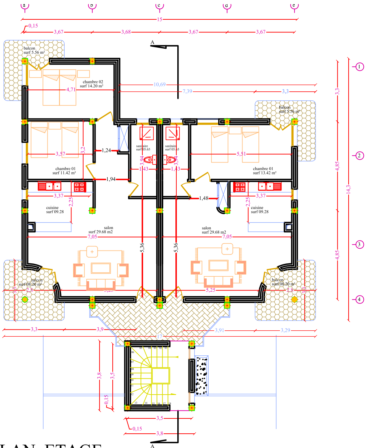
PLAN ETAGE
