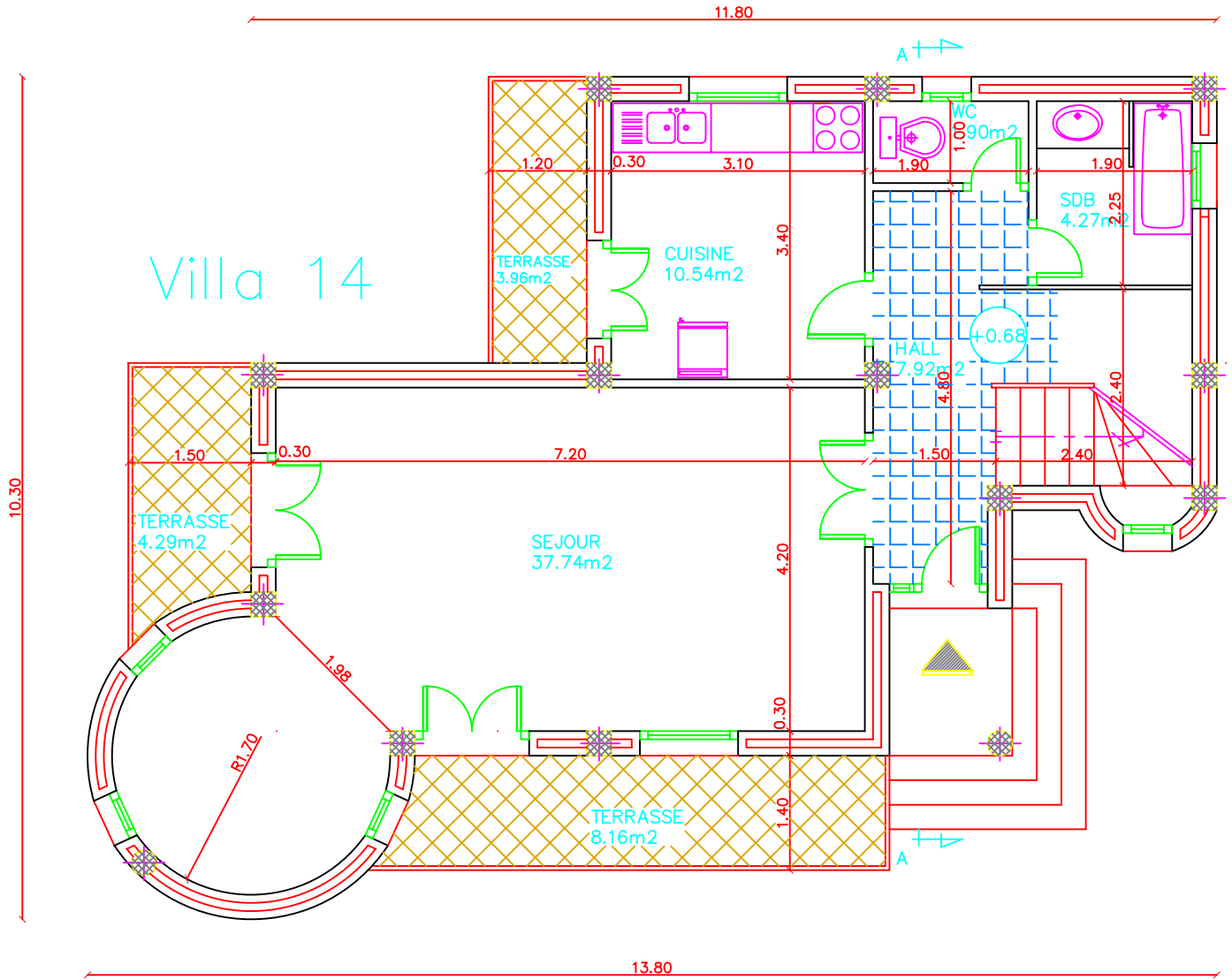
Vue en plan rez-de-chaussee
