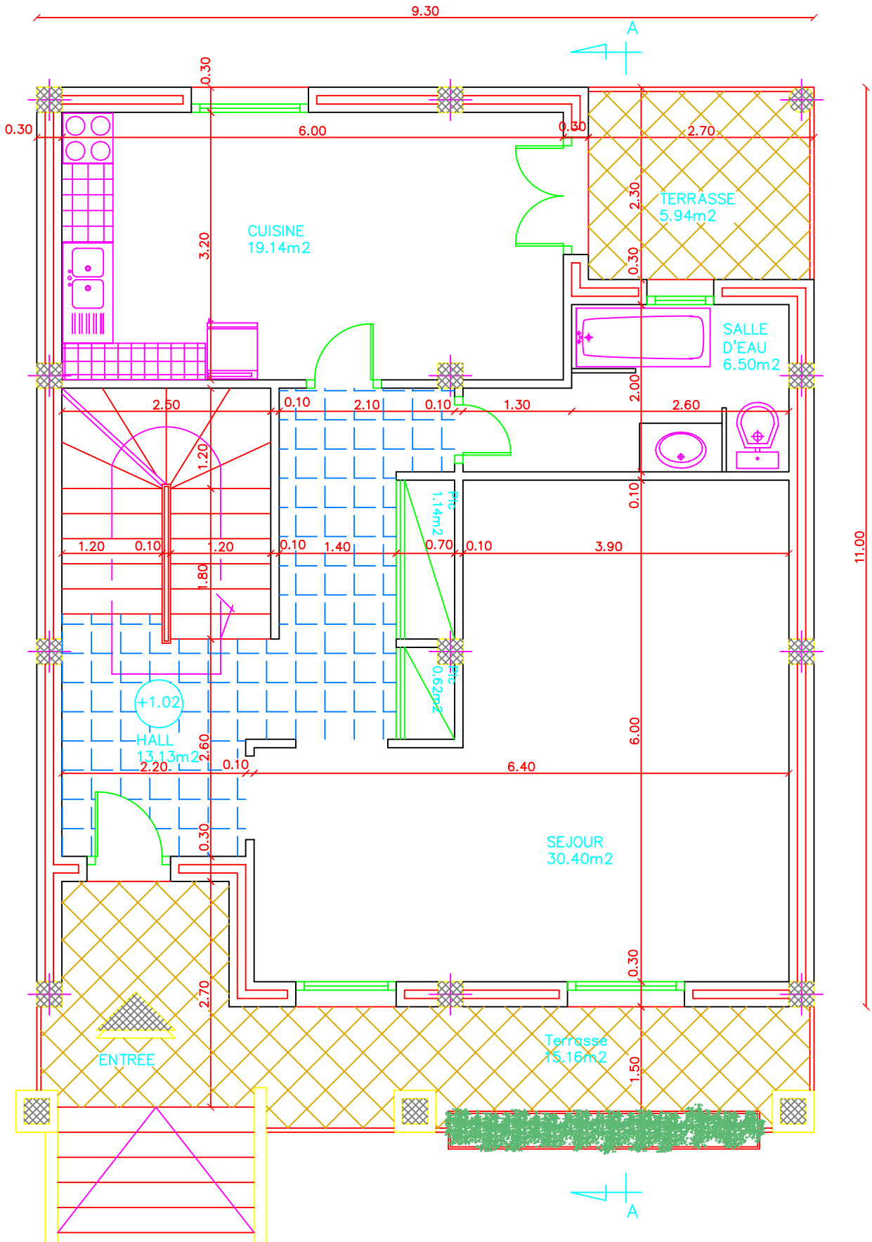
Vue en plan rez-de-chaussee
