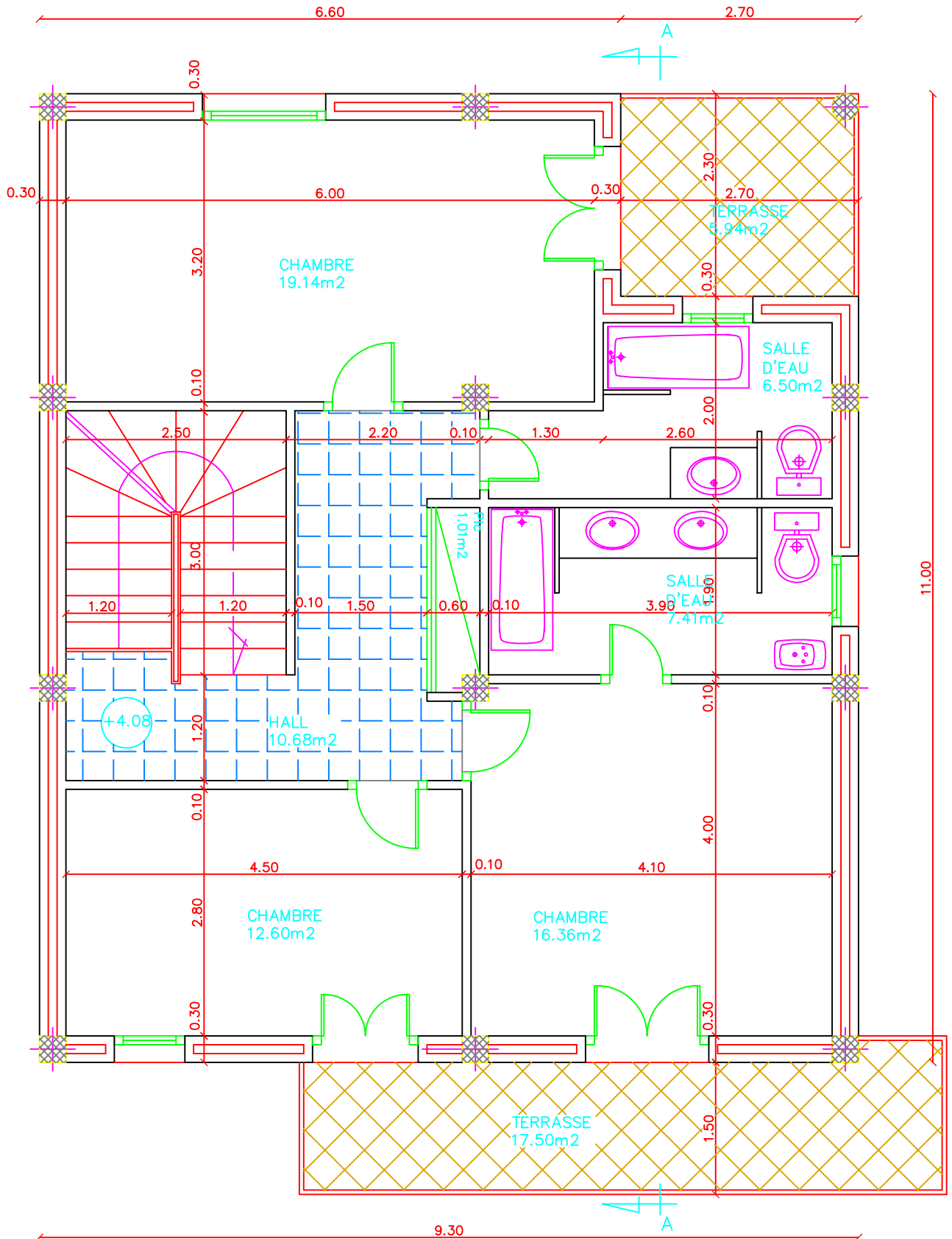
Vue en plan 1er Etage
