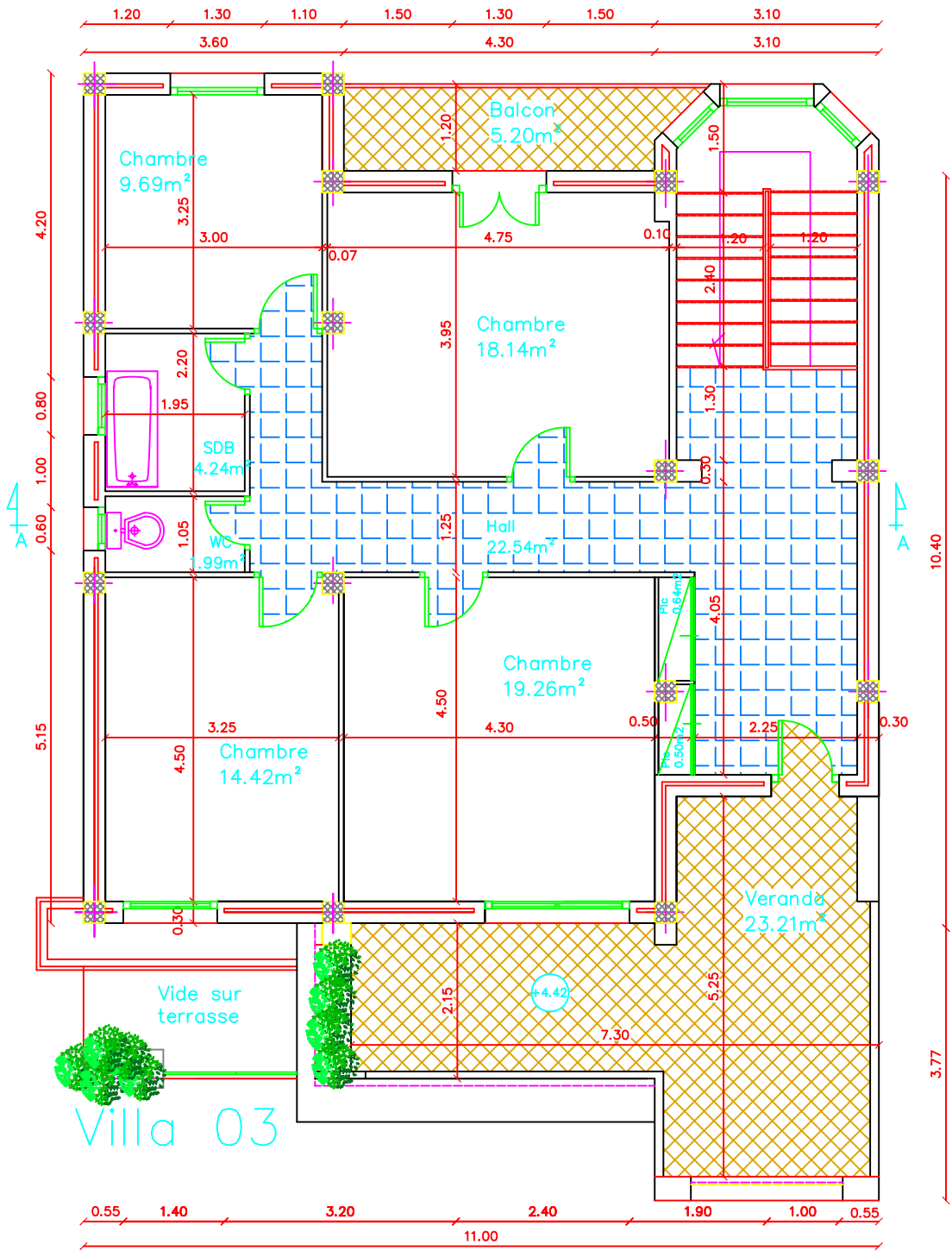
Vue en plan 1er Etage
