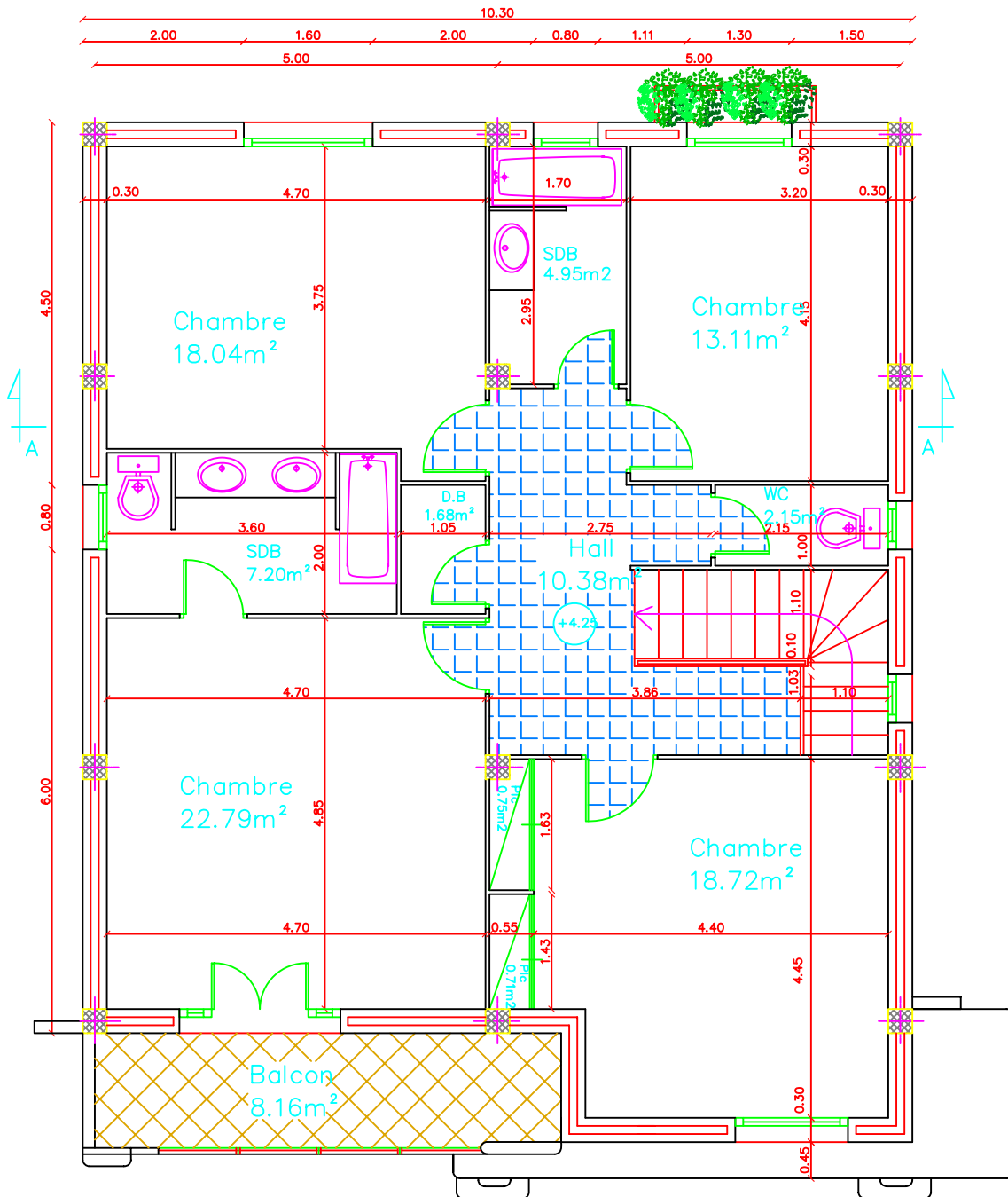
Vue en plan 1er Etage
