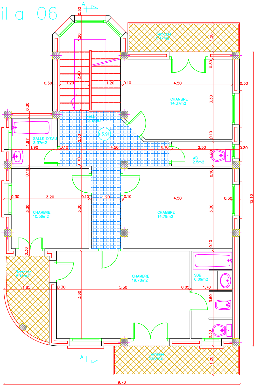
Vue en plan 1er Etage
